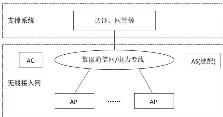
图 3.4.1 无线局域网基本结构图
